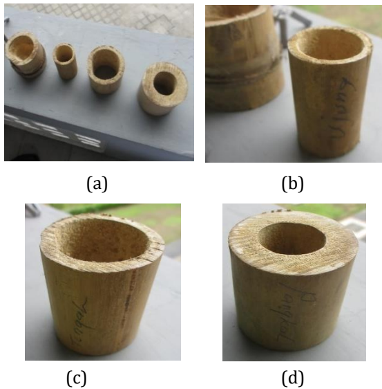
Gambar 2 Sampel Benda Uji Bambu Tali A) Tampak Keseluruhan, B) Bagian Ujung Batang, C) Bagian Tengah Batang, D) Bagian Pangkal Batang
