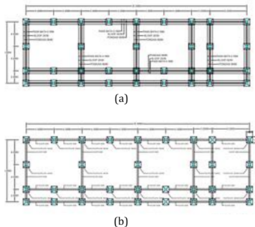
Gambar 2. Rencana Pondasi (a) Footplate dan (b) Sloof.
